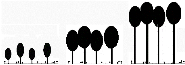
Figur 1. Energi från solen omvandlas i trädens blad till socker. Detta använder träden till att hålla liv i alla levande celler i krona, stam och rötter. Det kallas underhållsandning. Om det finns överskott på socker kan trädet använda det för tillverkning av ny ved, dvs. för tillväxt. Bladytan, som fångar solens strålar, är minst i ungskogen till vänster. Bladytan hos beståndet i mitten är tillräcklig för att fånga allt ljus. Bladytan kan inte bli större. När träden blir högre lyfts bladytan allt högre upp utan att produktionen av socker ökar. När stammarna blivit så långa, som i beståndet till höger, förbrukas en allt högre andel av sockret till andning i stammar, grenar och rötter. Då avtar tillväxten över tiden.
