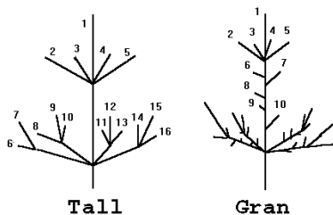
Figur 5.03. Frihetstal på tall är det antal nya skott som bildats ur toppknoppen för två år sedan. Frihetstal för gran är det antal nya skott som bildats på fjolårets toppskott. Antalet frihetstal skiftar hos tall från 1 till 70 och hos gran från 3 till 35, enligt mina egna observationer.
