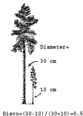
Figur 5.01.. Dissimilarity coefficient (Disco) är det absoluta värdet av skillnaden dividerat med summan. Talet beräknas för par av träd som står nära varandra. Coefficienten är 0.0 när alla träd är lika stora och 1.0 när maximal ojämnheter föreligger. När skogen är naturligt fullskiktad blir medeltalet av disco hos många par = 0.5. (Hagner och Nyqvist 1998)
