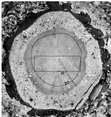
En plank på 50 x 150 mm har sågats efter märkeklyvning. Den innehåller enbart ungdomsved.
