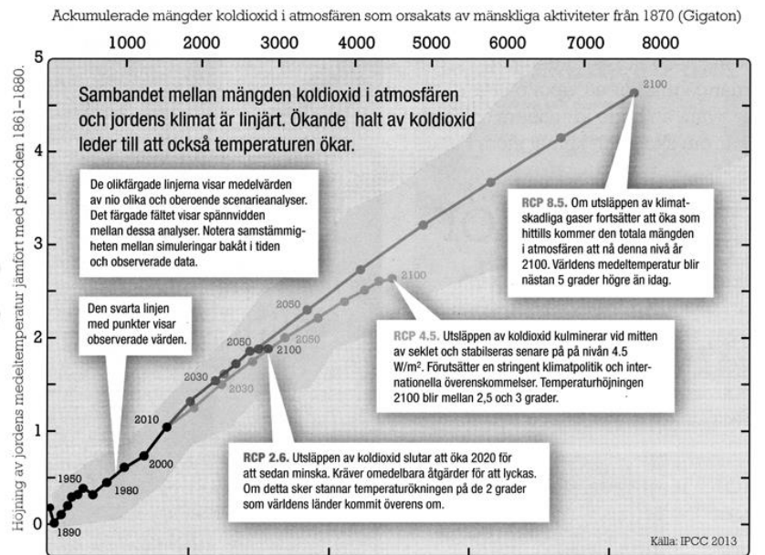
Figur 15.04. Om nuvarande utveckling av CO 2 -emission fortsätter, kommer Sverige att på sommaren år 2100 vara 5 grader varmare och ha 10-20 % mer nederbörd. Samtidigt kommer det i södra Europa vara 7-10 grader varmare och mycket torrare, - 30 % nederbörd (Bärring 2013).
