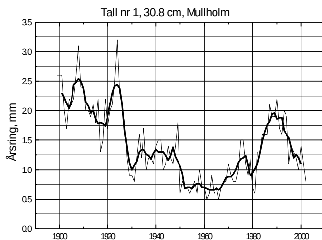
Figur 13.16. Årsringsutvecklingen hos en dominant tall nr 1 i (H). Brösthöjdsåldern är 105 år. Den grova linjen representerar fem års flytande medelvärde. Denna tall hade det allt svårare med konkurrenter fram till 1973 då höggallringen gjordes. Därefter har den successivt återhämtat sig till en kulmination på hela 2.0 mm 1990. Därefter drabbades den åter av ökande konkurrens, trots sin dominerande ställning i beståndet.
