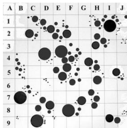
Figur 3.01. Ett skogsområde är indelat i 81 ytor med 2.5 m sida. De största träden har diametern 30 cm. Som i en naturlig skog finns det många småplantor och träden står mycket ojämnt utspridda.
