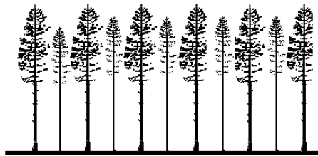
Figur 8.10. Särskilt vind- och snökänsliga är sådana träd som vuxit inklämnda mellan nästan likstora träd (Valinger och Lundqvist 1992). De får högt uppsatt krona och klen stam, s.k. "borstviskor". En typisk situation där träd får denna form, är i tät kulturskog med träd av ungefär samma längd. Vid befriande gallring skulle man föredra att befria de mindre kvalitetsdanade träden, men detta är ingen bra skötselmetod på grund av att dessa bryts ned av snö.
