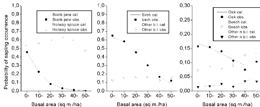
Figur 10.07. Sannolikheten att finna ett träd med 1-4 cm diameter i brösthöjd på en cirkelyta med 5 m radie (78 m 2 ) (Från Wikberg et al. 2004). Den vertikala axeln skildrar sannolikheten att det finns en eller fler träd av denna storlek. Den horisontala axeln skildrar beståndets täthet i grundyta per hektar. Underlaget för beräkningarna är hämtat från riksskogstaxeringen. Det framgår klart att de ljusälskande arterna tall och björk minskar i antal när bestånden blir täta medan de skuggfördragande arterna gran och bok är frekventa även där skogen är tät. Andra uppgifter i detta arbete är att barrträd av denna storlek uppträder på 66 % av alla ytor ( r=5m ) och att det i medeltal i Sveriges skog finns 99 tallar och 351 granar av denna storlek per hektar.
